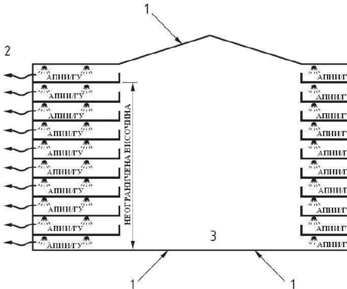
Фиг. 1. Строежи от клас на функционална пожарна опасност Ф4 и Ф5; атриум с височина над 25 m, отворен към съседните етажи.
